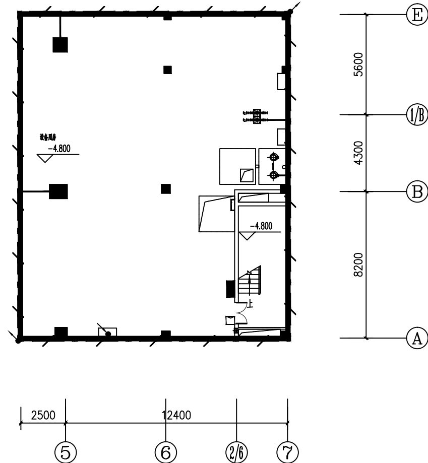
地下一层公共广播平面图 1:150
