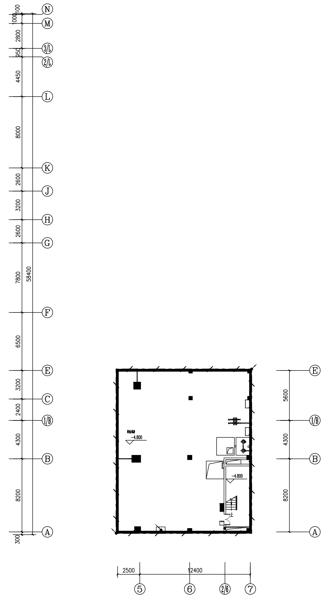
地下一层综合安防平面图 1:150
